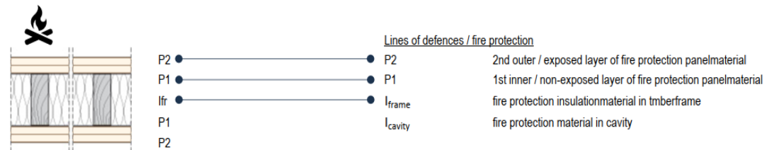
Figuur 1: De initiële bescherming (defense lines) van houtskeletbouwelementen door beschermend plaatmateriaal.
