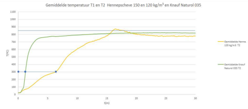
Gemiddelde temperaturen onderkant (T2) + Glaswolref.
