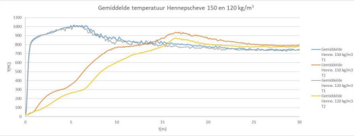
Gemiddelde temperaturen oppervlakte (T1) en onderkant (T2)
