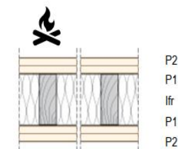
Figuur 7: Initiële bescherm lagen in een HSB-wand
