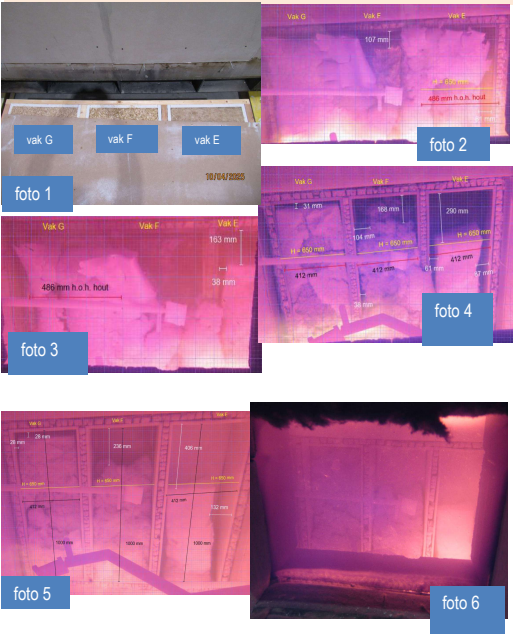
Waarneming tijdens test: Foto 1: Constructie vakvullingen (vanaf de vuurzijde) Foto 2: Constructie, wegvallen MDF na 18 minuten beproeving Foto 3: Constructie, wegvallen MDF na 20 minuten beproeving Foto 4: Constructie na 30 minuten beproeving Foto 5: Constructie na circa 60 minuten beproeving Foto 6: Constructie na 90 minuten beproeving
