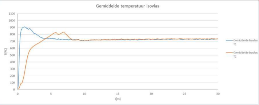
Gemiddelde temperaturen oppervlakte (T1) en onderkant (T2)
